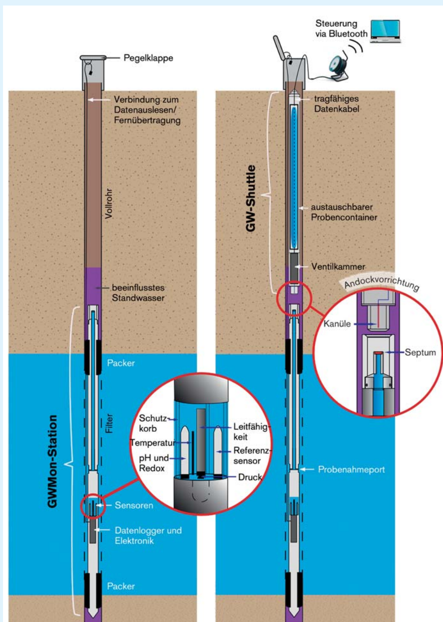
FUNKTIONSPRINZIP: GWMon-Station im stationären Monitoringbetrieb (links) und Probenahme mit dem GW-Shuttle (rechts)
