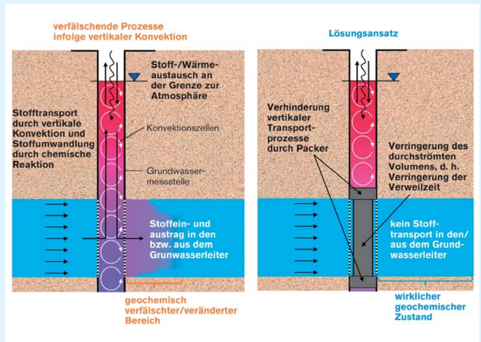
PROBLEM UND LÖSUNG: Konvektive Stoff- und Wärmeflüsse in Messstelle und Grundwasserleiter und deren Verhinderung Grafik: DGFZ
